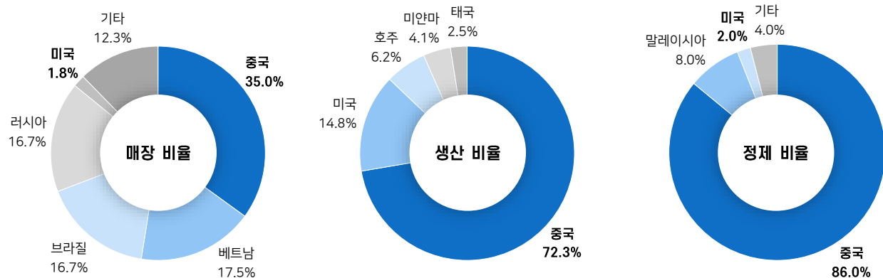
그림3 국가별 희토류 매장/생산/정제 비율
