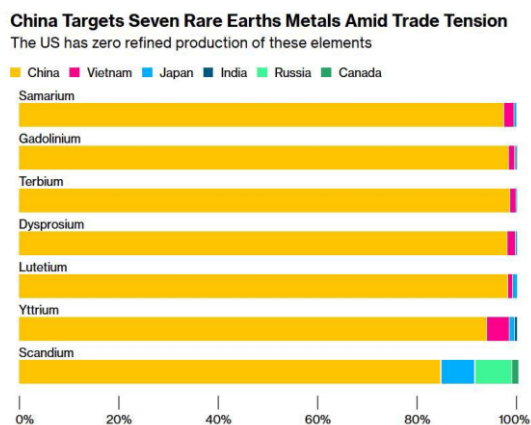
그림4 국가별 중희토류 정제 점유율
